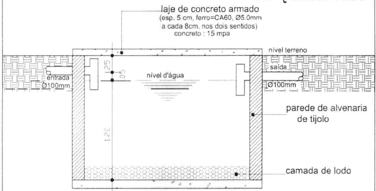
CORTE-AB
