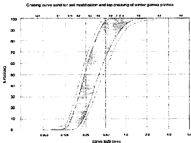
Curva de seleção para seleção de areia
