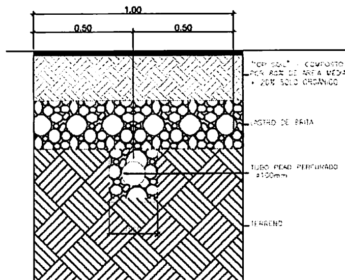
Figura 2 – Detalhe do Sistema de drenagem
