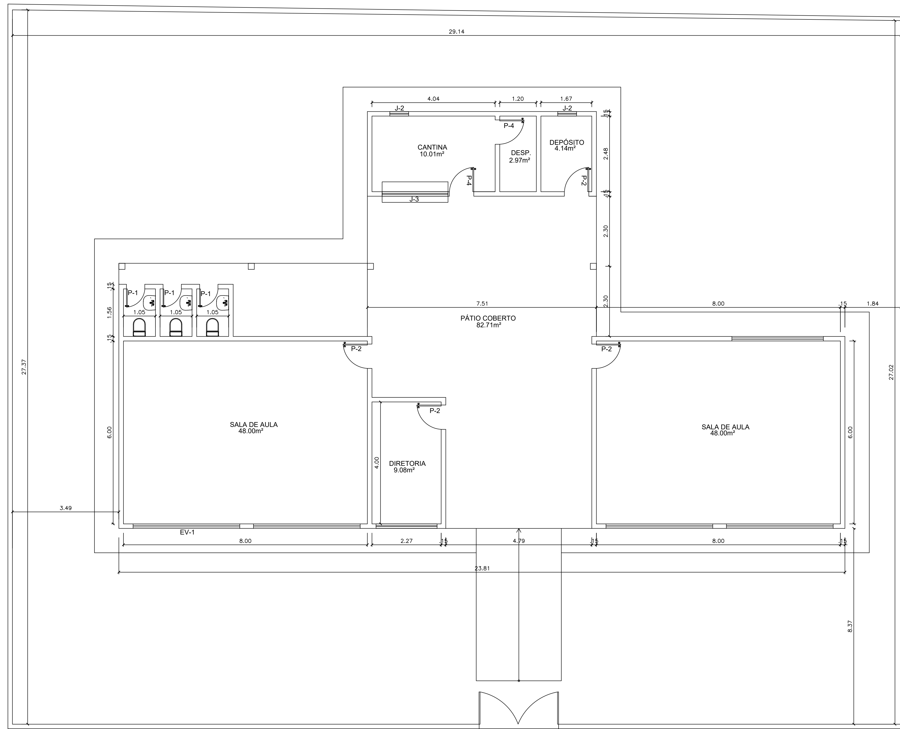
PLANTA BAIXA
